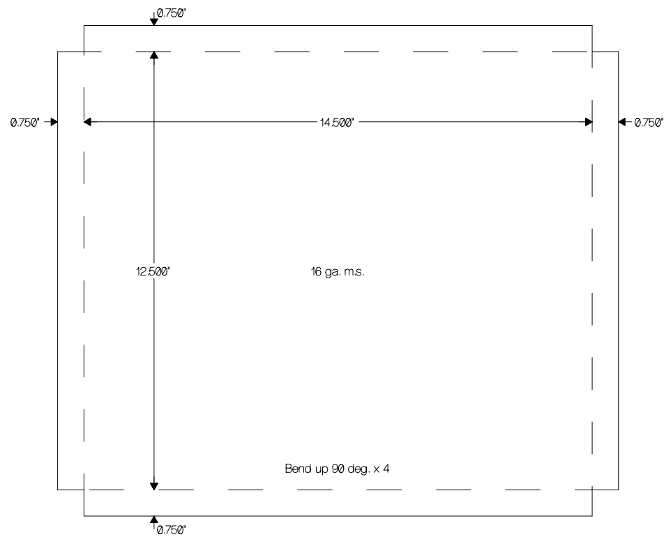
Lid Layout
